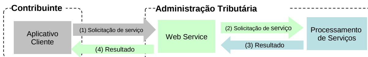
Figura 4-2 – Serviço de Implementação Síncrona
